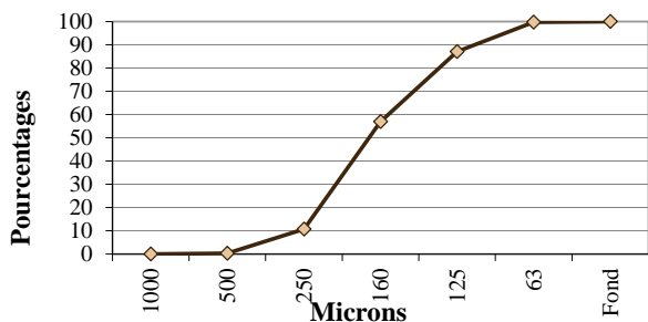
Courbe des refus cumulés (ASTM)
